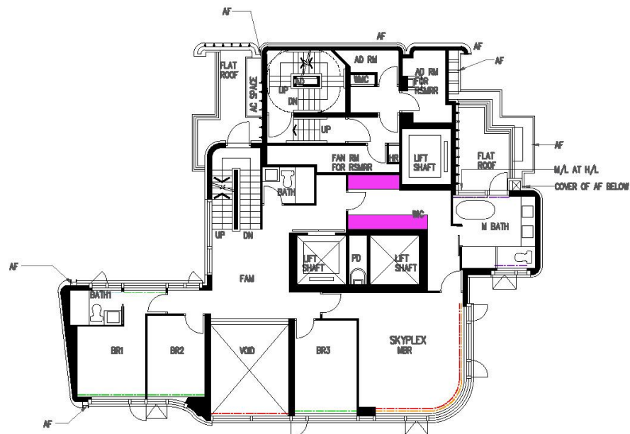
Tower 6 28/F Floor Plan 第6座 28樓平面圖
